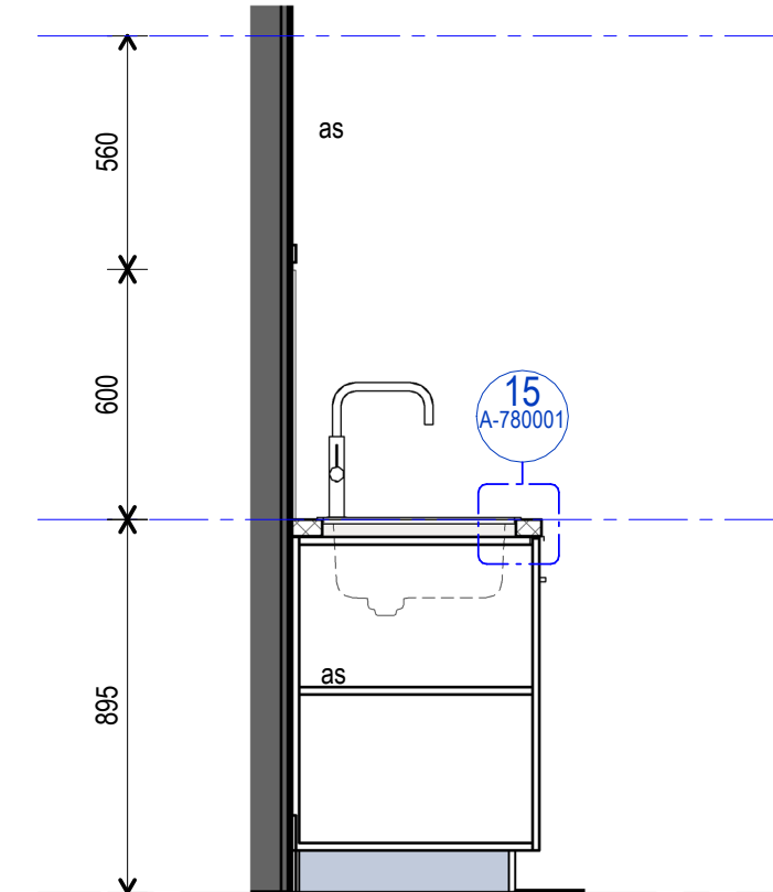
5 JO-BW-2 Section 2 1:20
