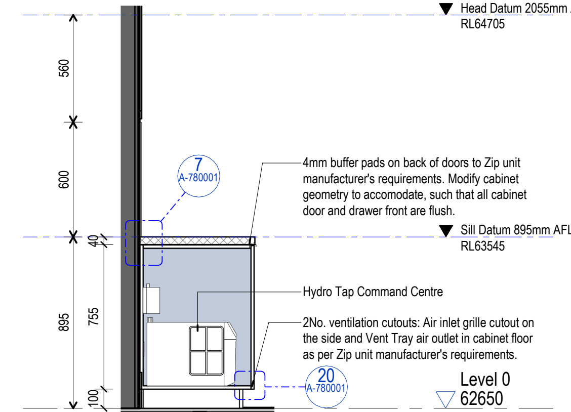
7 JO-BW-2 Section 1 1:20
