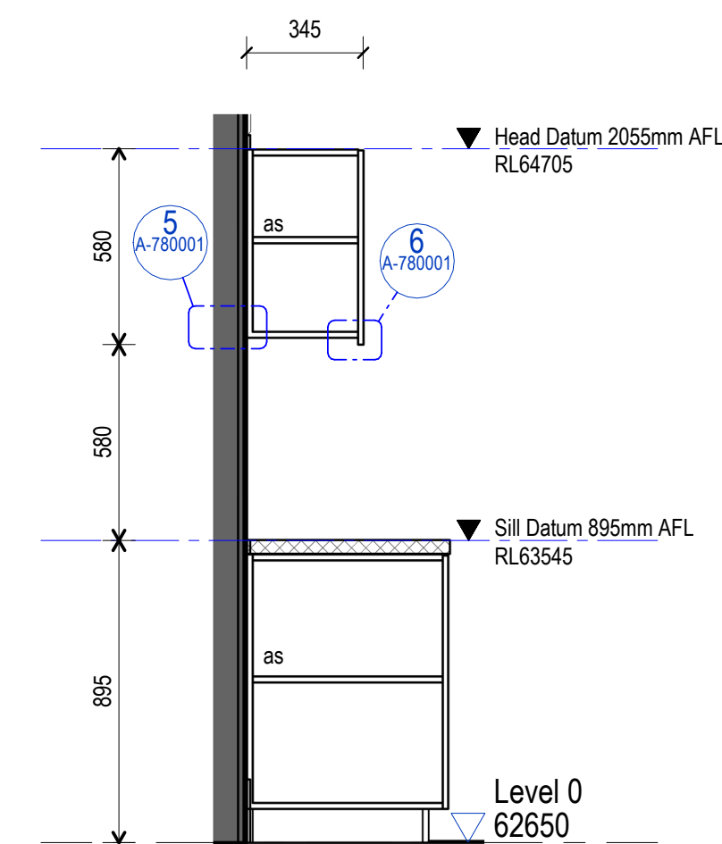
8 JO-BW-2 Section 2 1:20
