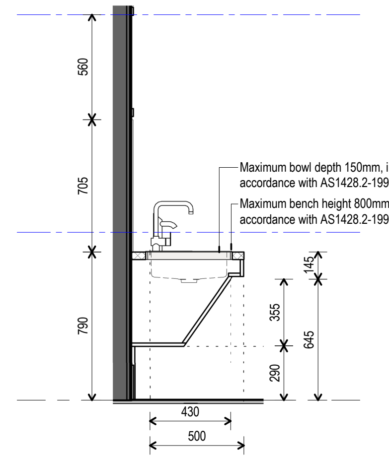
4 JO-BW-2 Section 1 1:20
