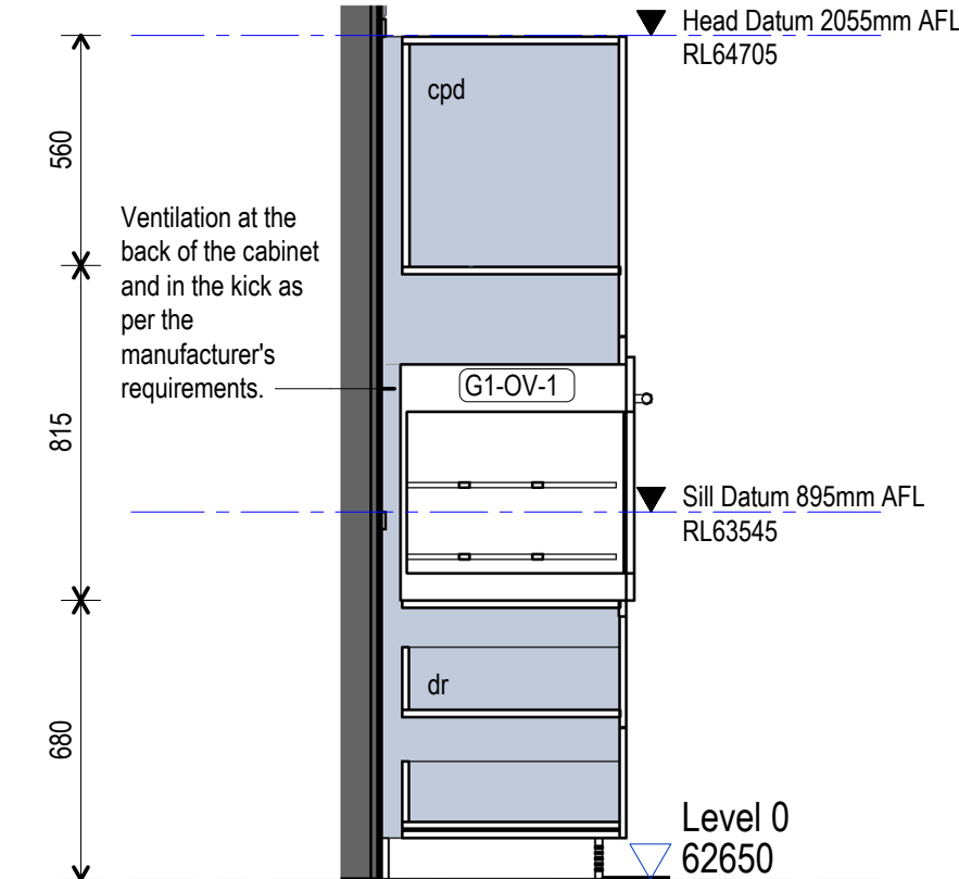
6 JO-BW-2 Section 2 1:20
